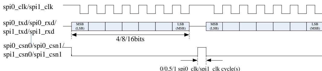
Fig. 20-4 SPI Format (SCPH=0 SCPOL=1)
