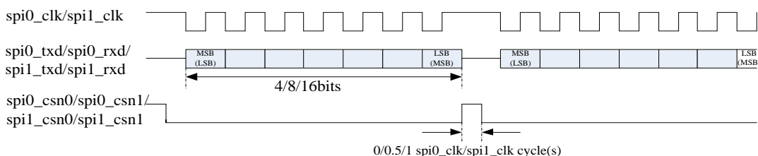
Fig. 20-6 SPI Format (SCPH=1 SCPOL=1)
